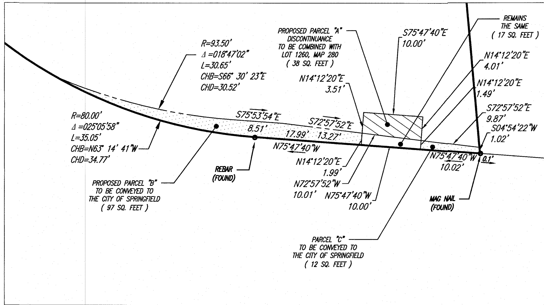
DETAIL "A" SCALE: 1" = 10'
